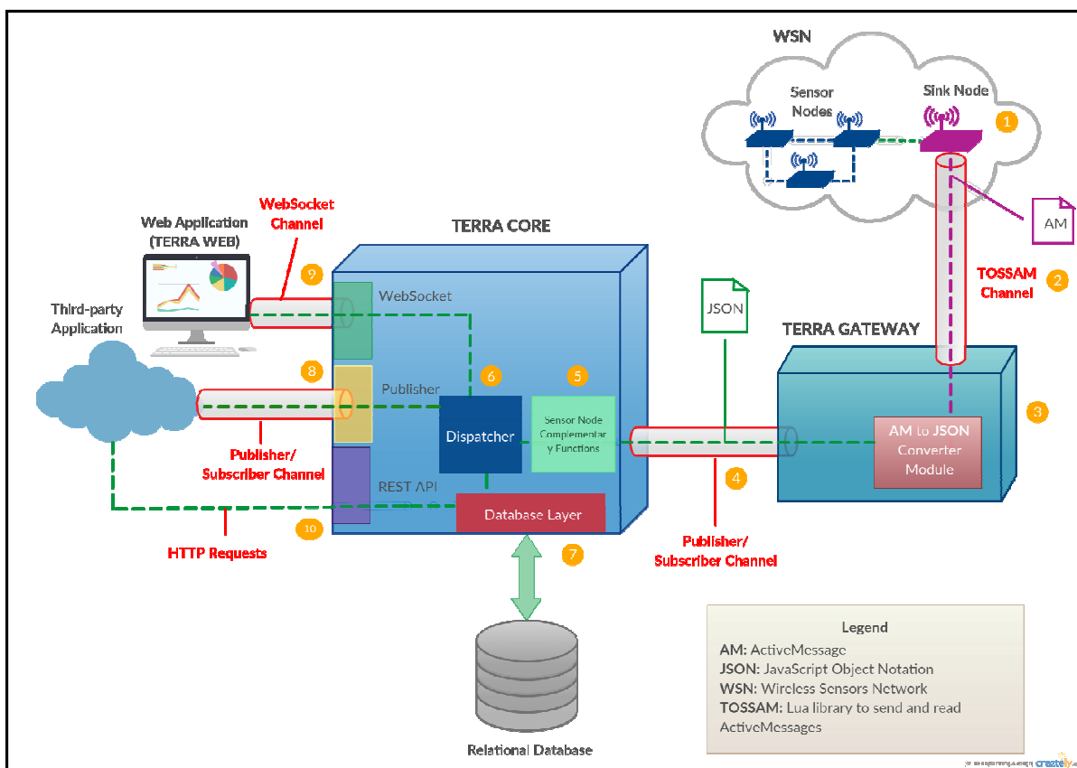
Figura 1. Visão geral da arquitetura e aplicações propostas
